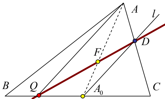
Рис. 25: до 1-го способу розв'язання задачі 4
